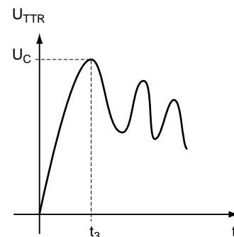
Fig. 7 : tension transitoire de rétablissement - TTR - assignée en cas de court-circuit aux bornes d'un disjoncteur (§ 4.102 de la norme CEI 60056).
